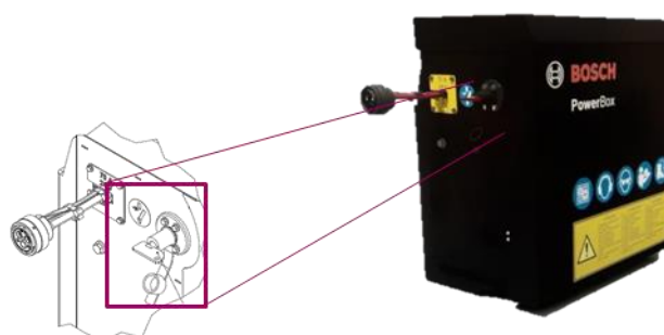
Figura 226 - Chave geral PowerBox
