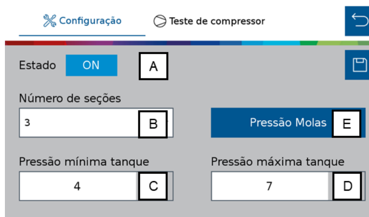
Figura 66 - Tela de configuração de molas pneumáticas
