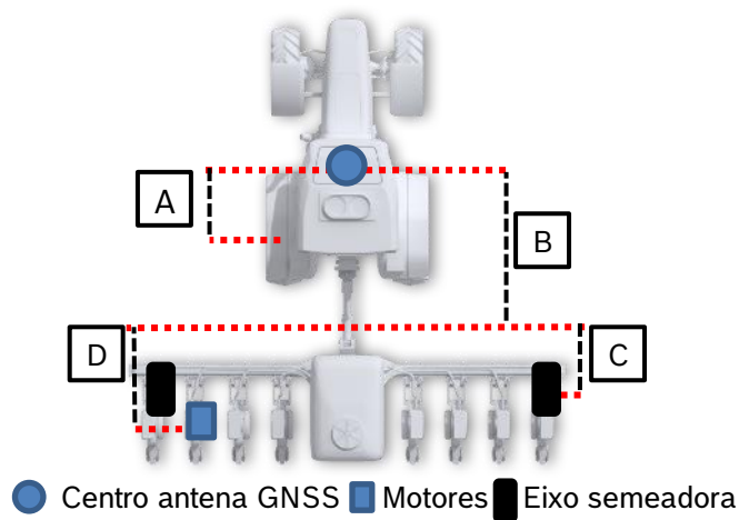
Figura 5 - Visualização das dimensões do trator
