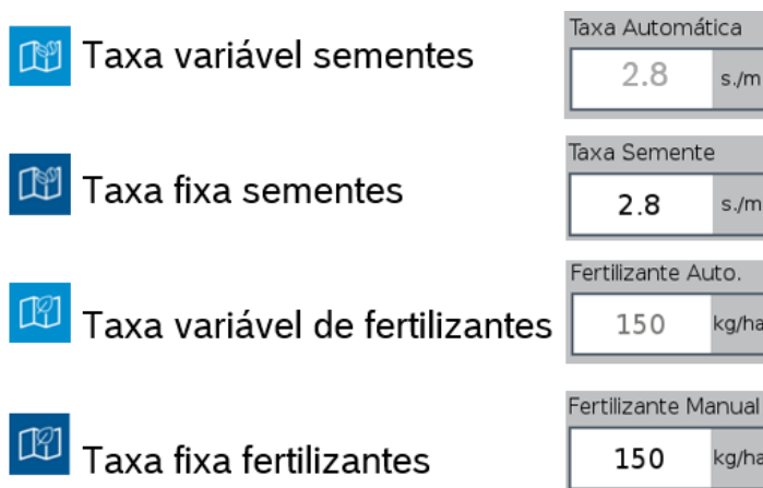
Figura 222 - Visualização taxa variável e taxa fixa
