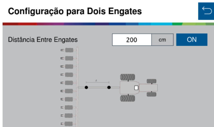
Figura 11 - Tela de configuração para Duplo Engates
