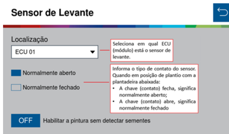
Figura 31 - Tela de configuração do sensor de levante
